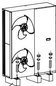
Podkładka antywibracyjna
