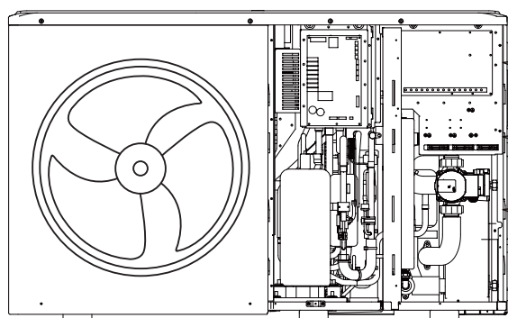
Układ chłodziwa
