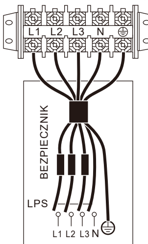
ZASILACZ JEDNOSTKI 3 fazy
